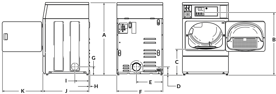
SDC10 pohľad z boku SDC10 pohľad zozadu SDC10 pohľad spredu
