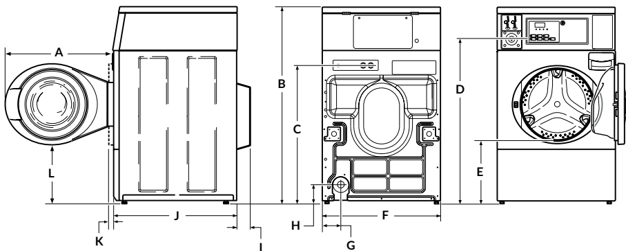
SPC10 pohľad z boku SPC10 pohľad zozadu SPC10 pohľad spredu
